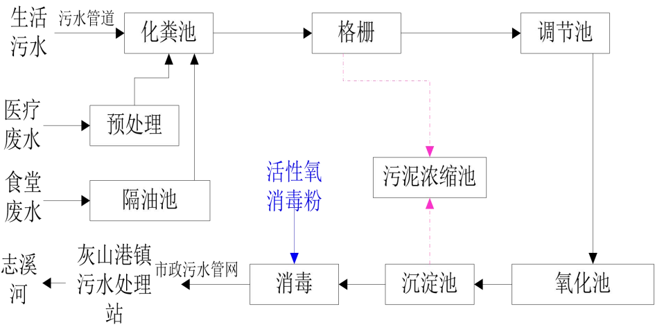
图 4-1 院内污水处理站工艺流程图
